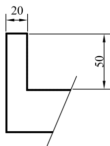
alzatina A2 standard
